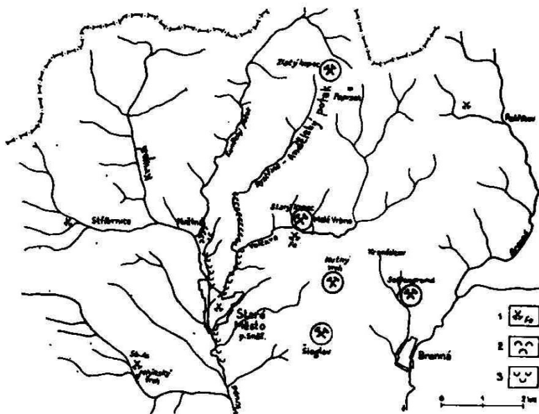
Pozůstatky po těžbě rud na Staroměstsku: 1 - staré báňské práce s označením zjištěné rudy, 2 - stará rýžoviště existující, 3 - stará rýžoviště aplanovaná a rekultivovaná
