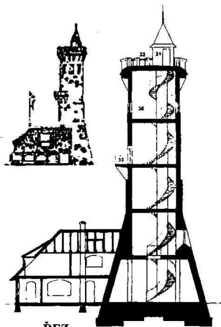
ŘEZ
